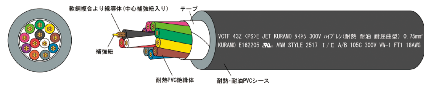
構造略図
