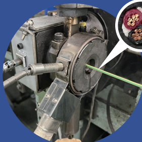
ぜつえんおしだし 絶縁押出工程
