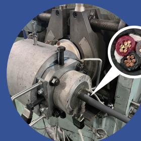
おしだし シース押出工程
